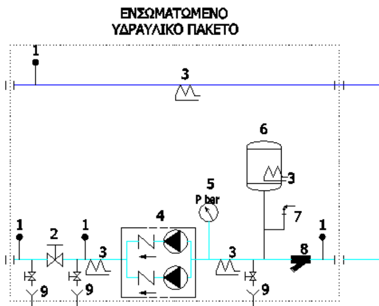
Σχέδιο 2 . Υδραυλικό συγκρότημα
